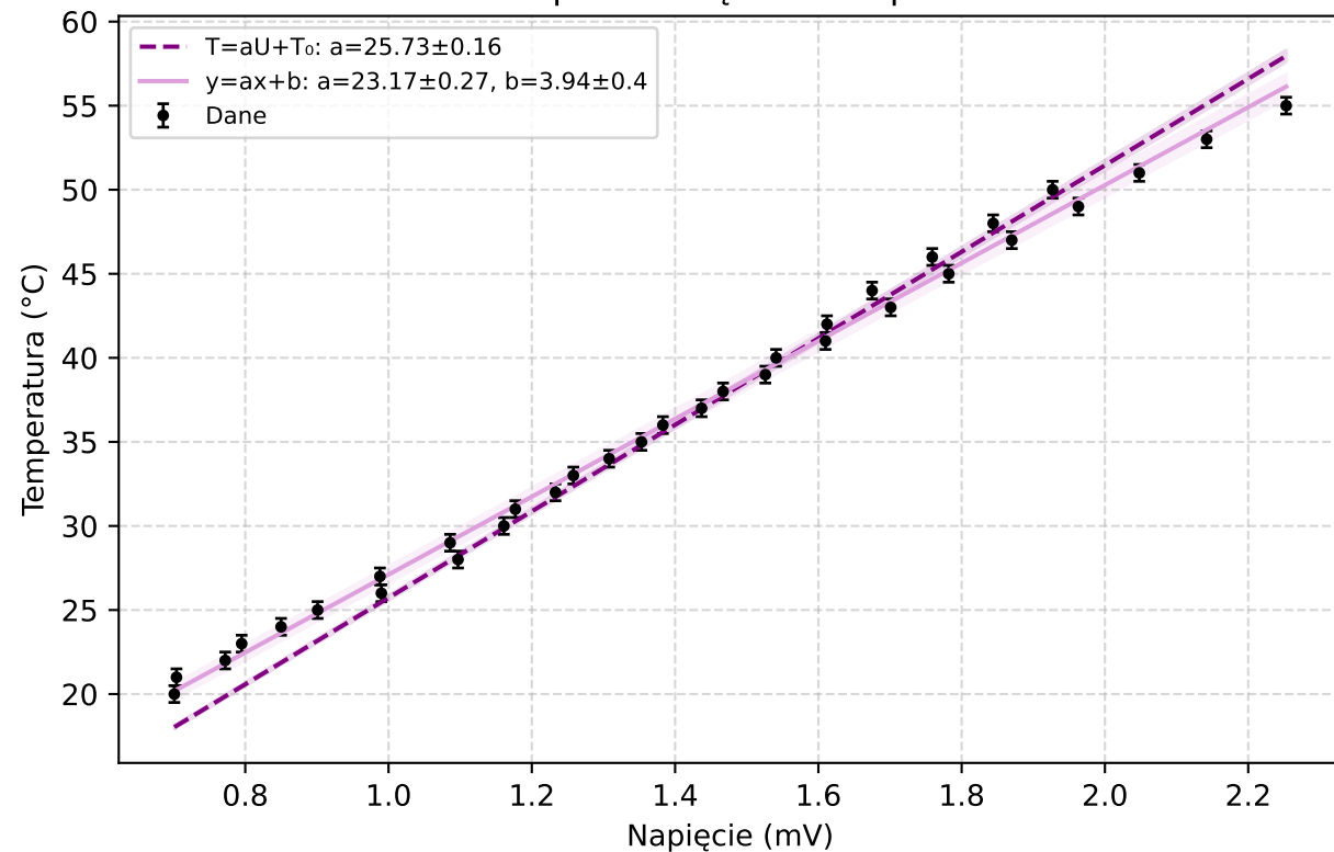
Termopara — Łączone 1. połowa
